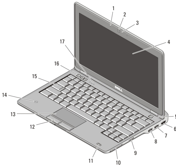
1. ábra. Előlnézet
